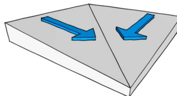
Kehlplatte (einteilig)
